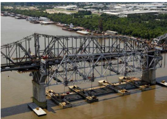
图 1: Huey P. Long Bridge, 密西西比河
